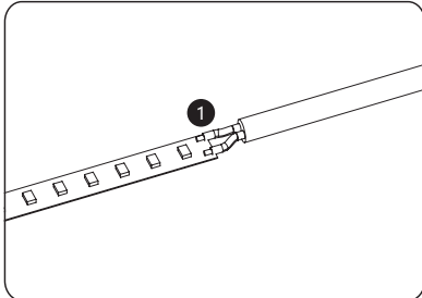
①. 将线与 PCB 板焊接起来;
