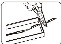
04 剪切模组到所需的数量，并把剪断后的线头做好防水和绝缘处理。 △ 注意：剪切模组间的导线时，请居中剪切
