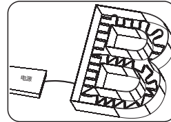
06 把模组正负极与电源输出端正负极正确连接。 △ 注意：线头做好绝缘、防水和防腐蚀处理，并以徒手不能拔掉为宜！
