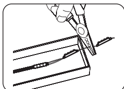
04 剪切模组到所需的数量，并把剪切后的线头做好防水和绝缘处理。 △ 注意：剪切模组间的导线时，请居中剪切
