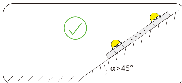
钝角斜面应用
