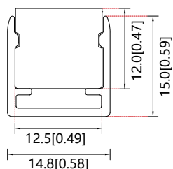
霓虹 + 型材后截面示意图：
