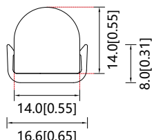
塑胶安装卡 型号: ASY-NDR1414-P1NNXXXX-MT
