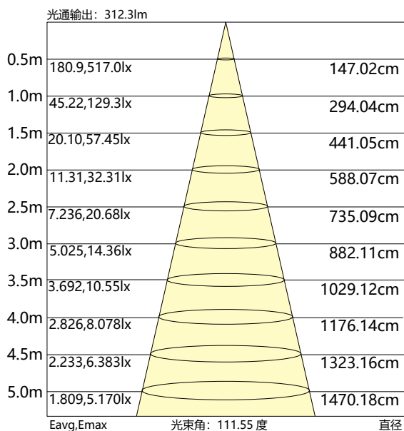
平均照度图
