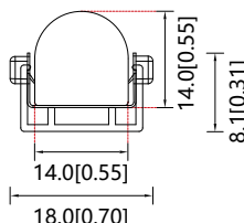
带金属弹片安装铝槽 型号: ASY-NDR1414-A2(A4)NNXXXX-MT
