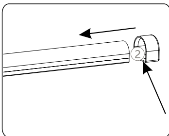
①. 堵头内部打上适量胶水，再推入灯带；②. 抹去多余胶水，待胶凝固，即可；
