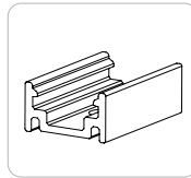
铝卡（选配） 数量（10米）： 型号：ASY-NDR1010-A3NN0020-MT 订购号：01.08.04221110010020 尺寸：20*7*13mm
