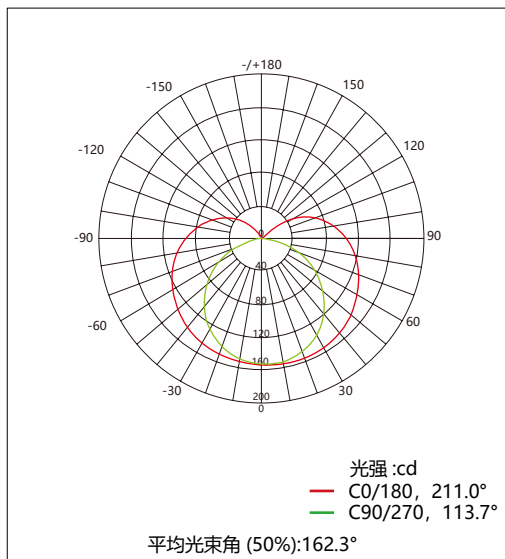
配光曲线
