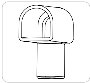
有孔堵头（下出）（选配） 数量（10米）： 型号：ASY-NDR1010-N00NNB-EC 订购号：01.06.KL23041701 尺寸：18*12*24mm
